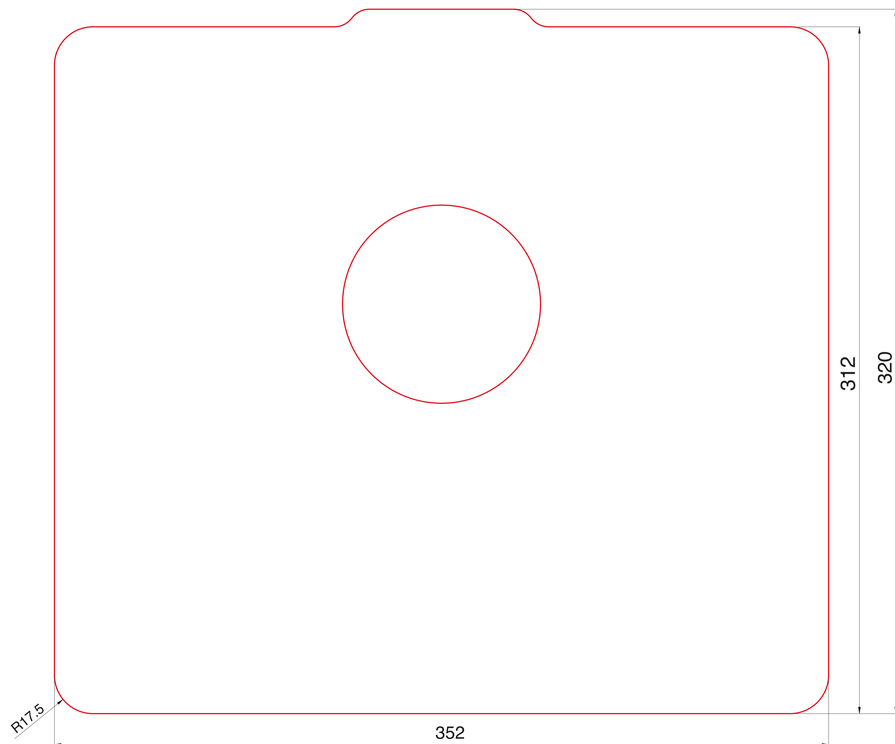
Dimensões para desenvolvimento da faca de corte
